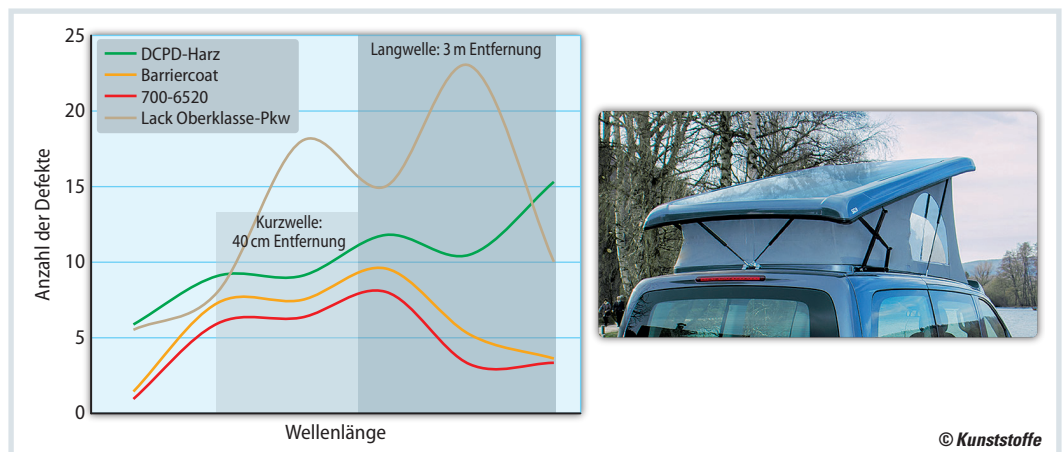
Bild 2. Für hohe Oberflächenqualitäten im RTM-Verfahren: Qualitätsvergleich aus WaveScan-Messungen (links). Für SCA-Dächer verschiedener Fahrzeughersteller setzt C. F. Maier das BÜFA-Resin VE 6520 im RTM-Light-Prozess ein (rechts) (© links: Courtesy of BYK-Gardner, rechts: C.F. Maier)
